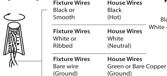
Fig. 2 Wiring
